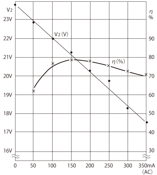
MG41-01出力特性
