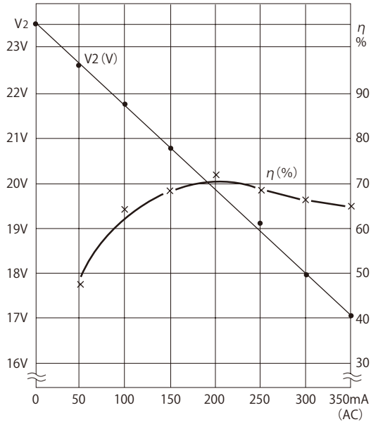
MU41-01出力特性
