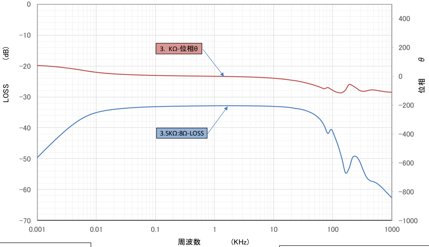
A86-35K08SA N01 周波数特性表
