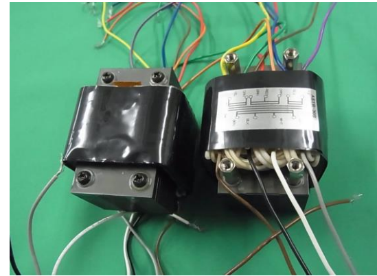
76) U II 型トランス例
