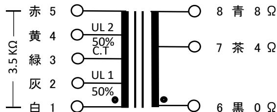
接続図
