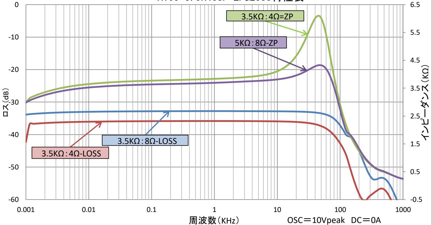
A105-3.5K48UP-ZP&LOSS特性表
