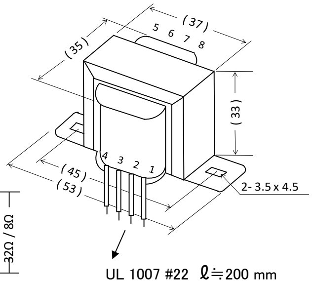
外形寸法図
