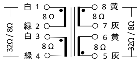
接続図
