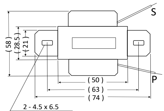
外形寸法図
