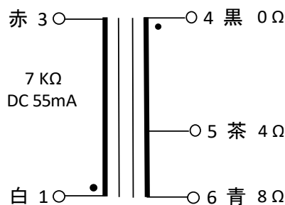
接続図
