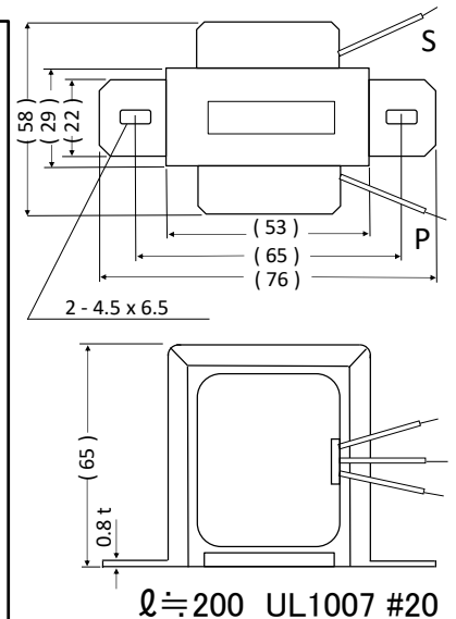
外形寸法図
