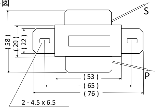
外形図
