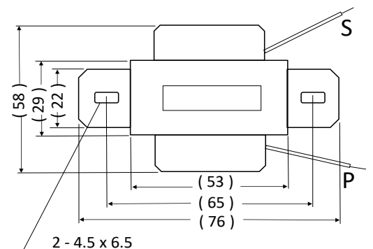
外形寸法図
