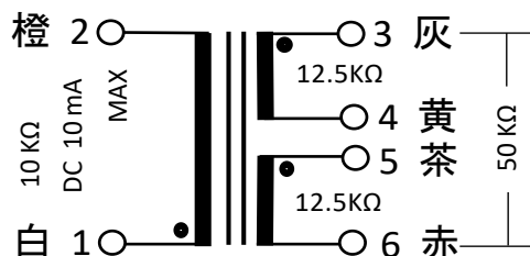
接続図
