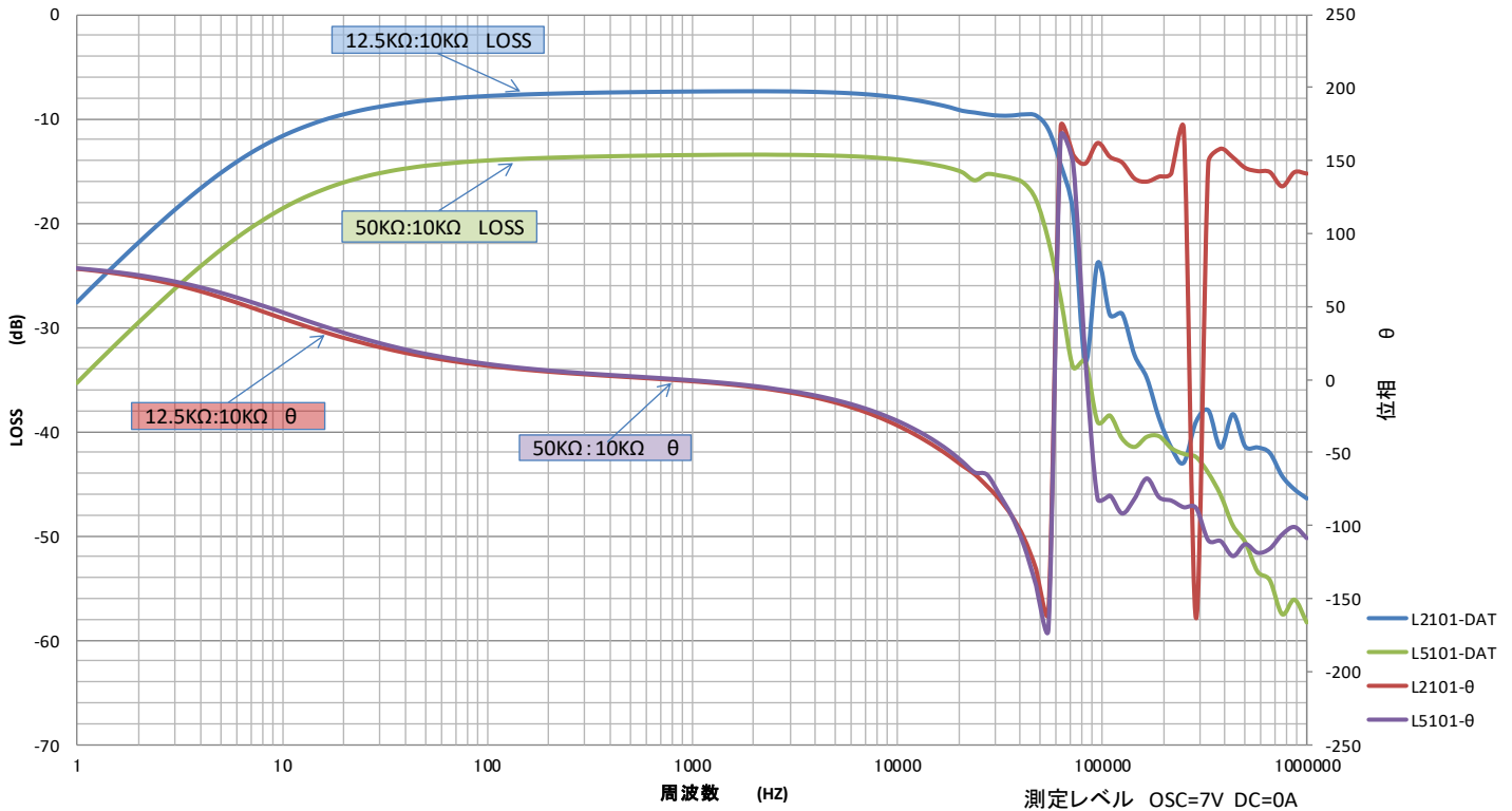
A60-10K125W N01 周波数特性表
