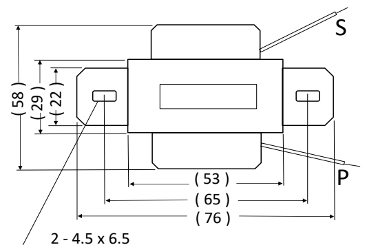
外形寸法図
