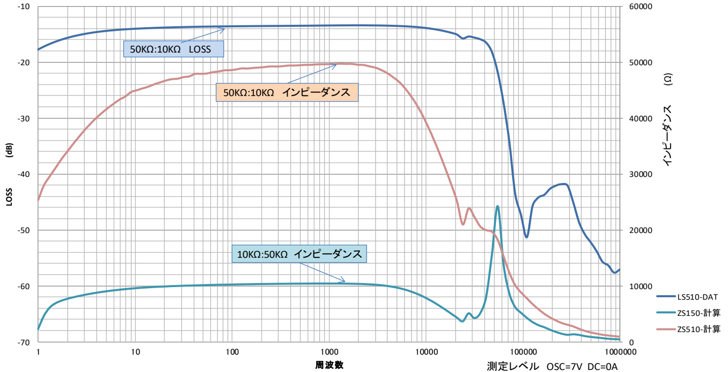
A60-10K50 N01 周波数特性表
