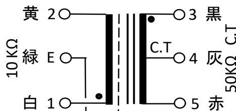
接続図
