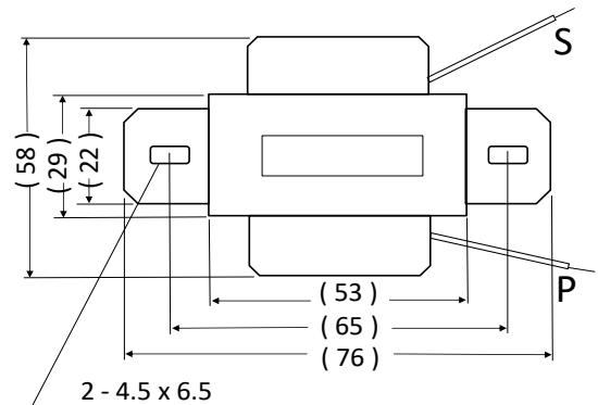
外形寸法図
