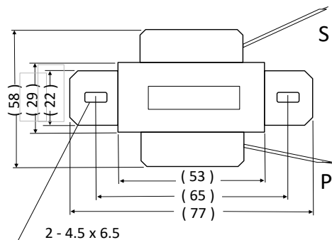
外形寸法図
