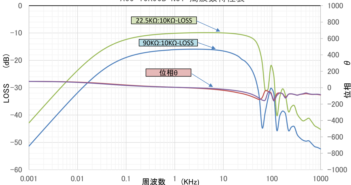
A60-10K90B N01 周波数特性表
