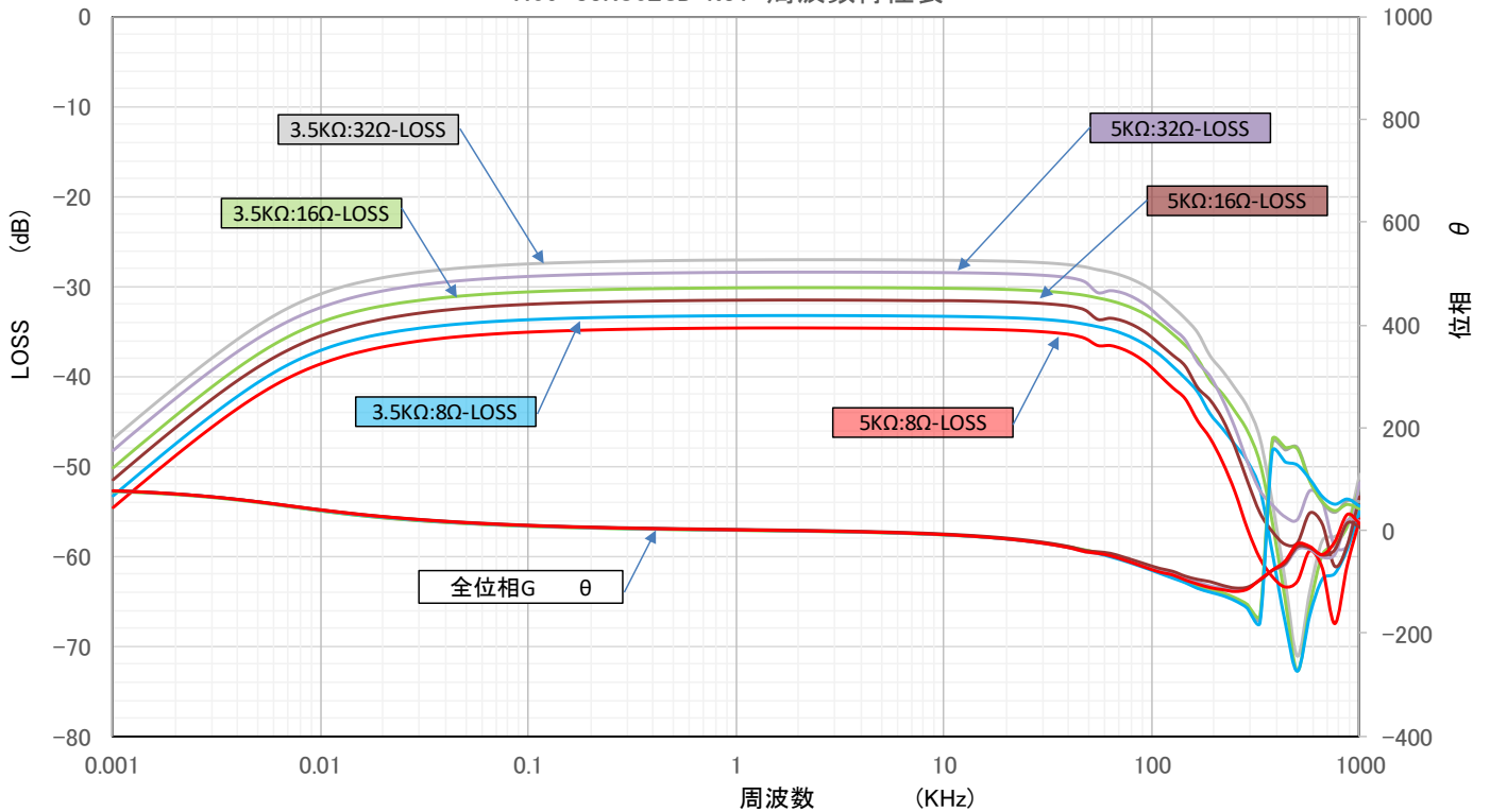
A60-35K862SB N01 周波数特性表
