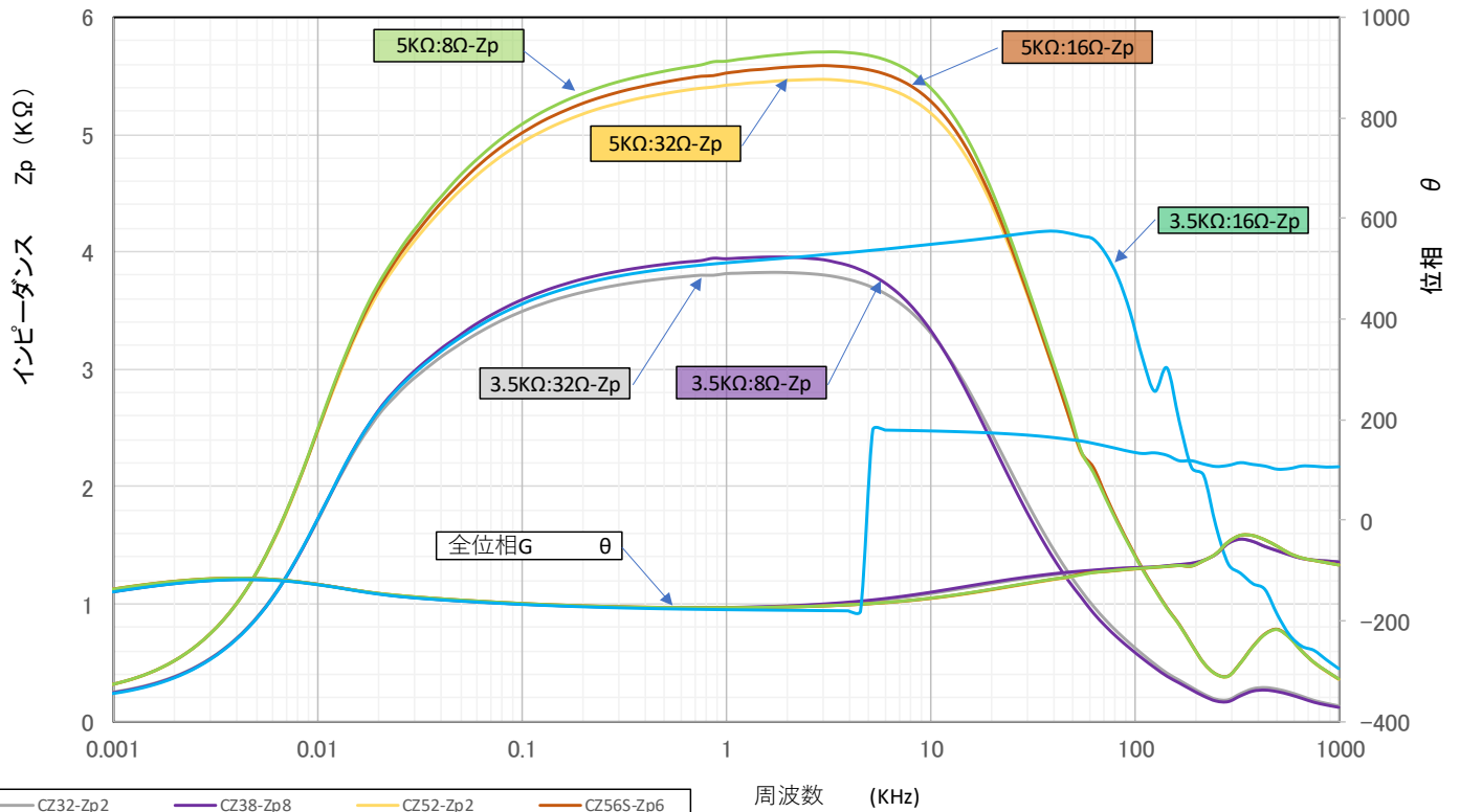
A60-35K862SC N01 インピーダンス特性表
