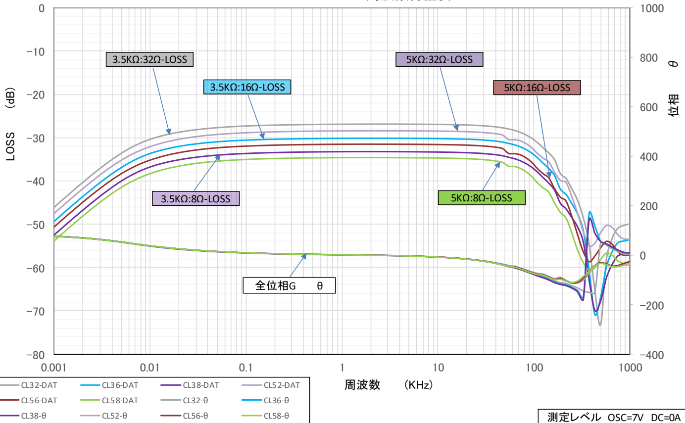
A60-35K862SC N01 周波数特性表
