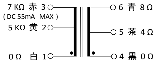
接続図
