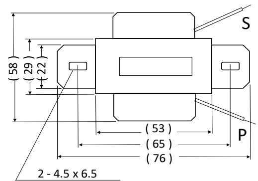
外形寸法図
