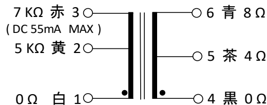
接続図
