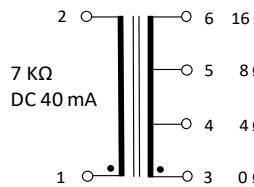
接続図
