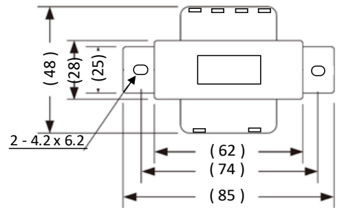
外形寸法図
