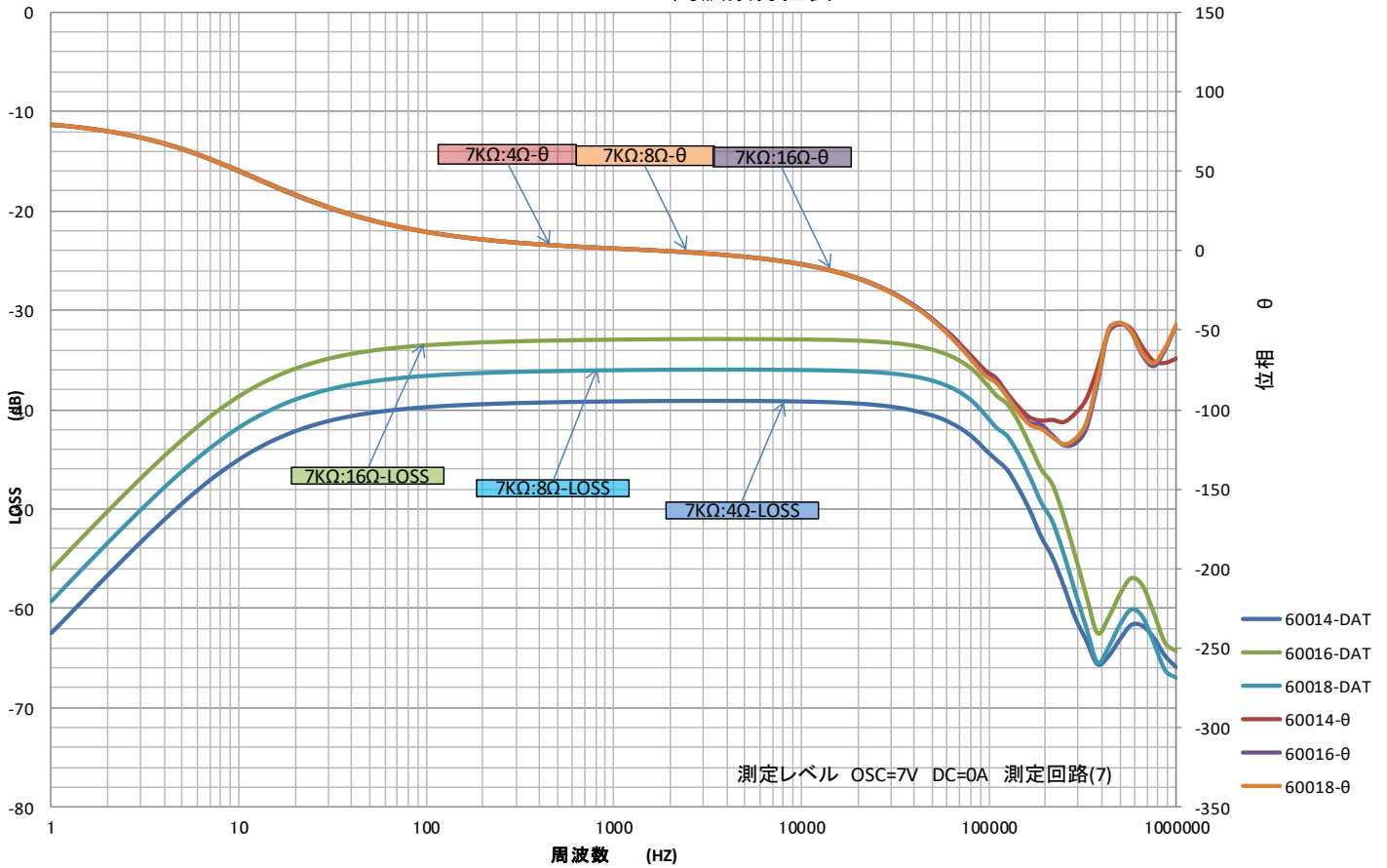
A60-7K4816S N01 周波数特性表
