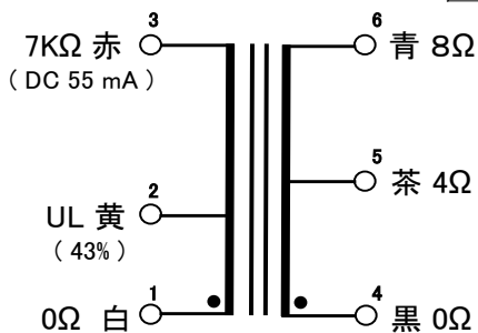
接続図
