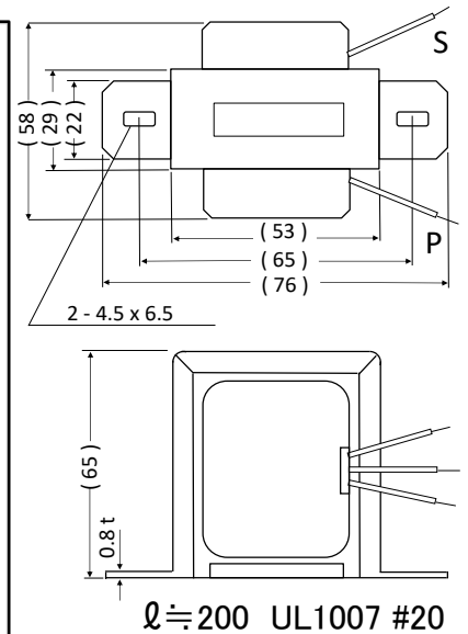
外形寸法図
