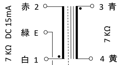
接続図
