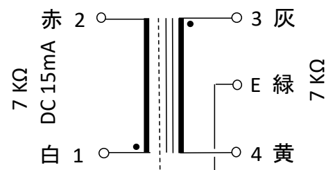
接続図
