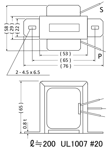
外形寸法図
