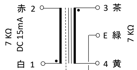
接続図
