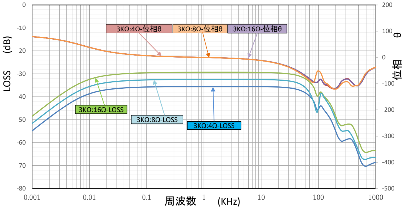
A66-3K486ST N01 周波数特性表
