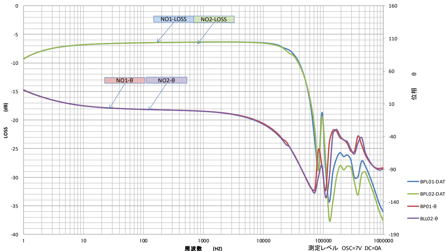
A76-10K10BP NO1 NO2 周波数特性表
