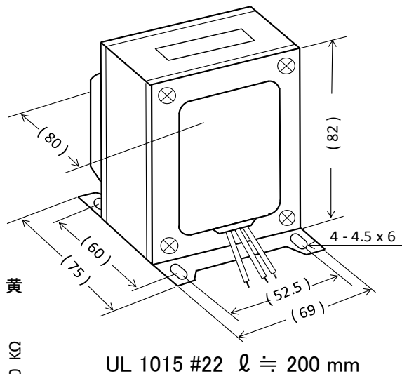
外形寸法図
