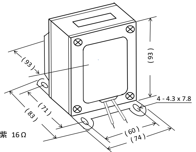
外形寸法図
