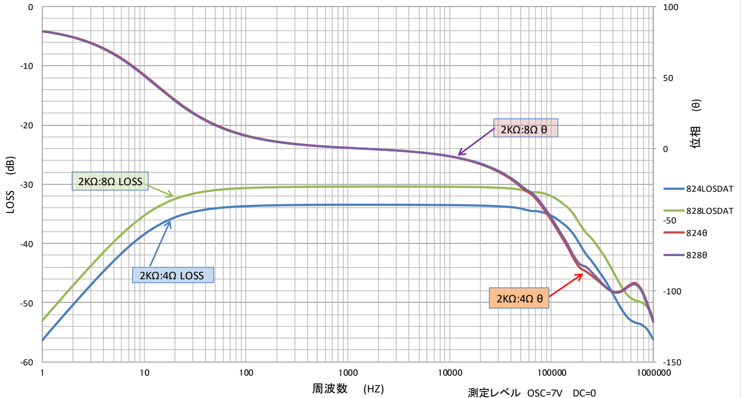
A86-2K48S 周波数 位相特性
