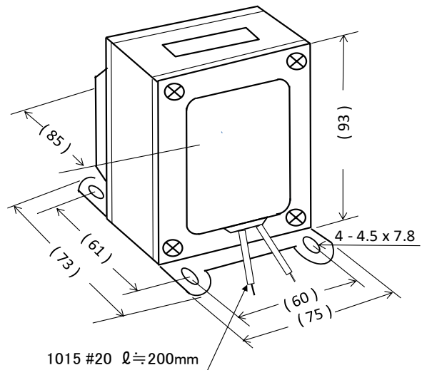
外形寸法図
