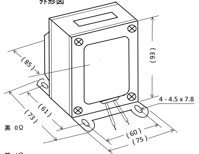
外形図
