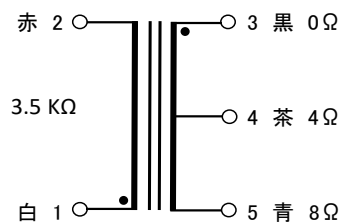
接続図
