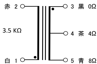
接続図
