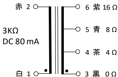
接続図
