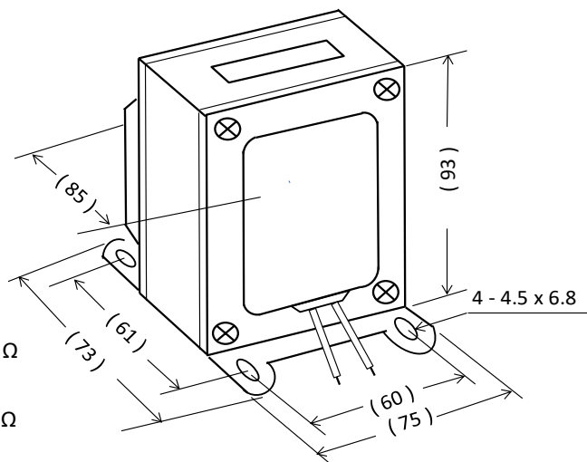
外形図
