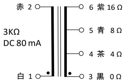
接続図
