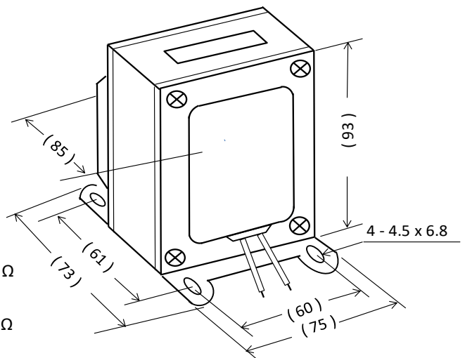
外形図
