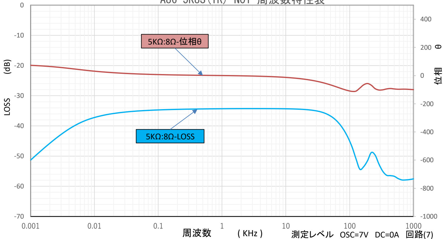
A86-5K8S (TR) N01 周波数特性表
