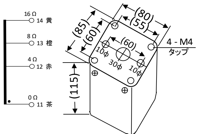
外形略図
