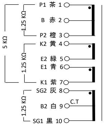
接続図
