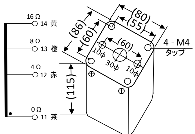
外形略図
