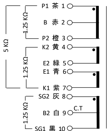
接続図
