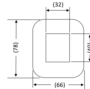
外形寸法図
