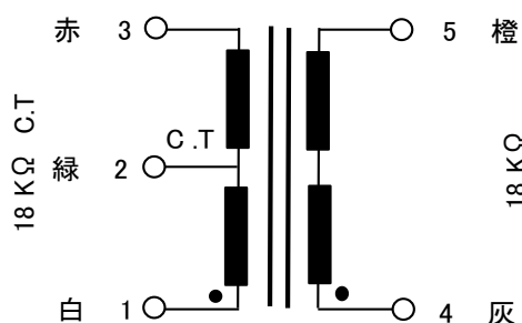
接続図
