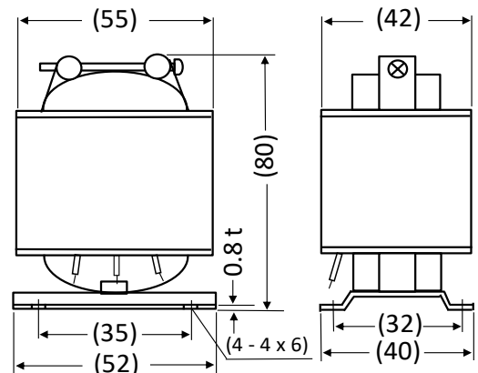
外形寸法図
