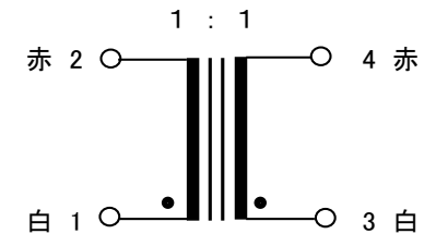
接続図
