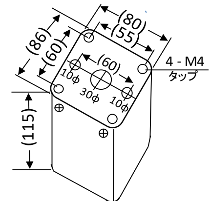
外形寸法図
