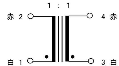
接続図
