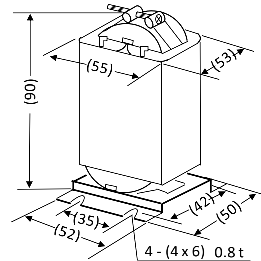
外形寸法図
