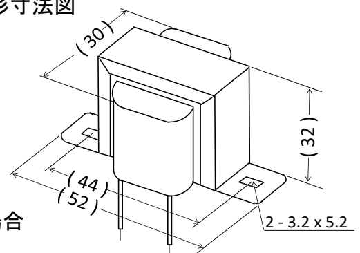
外形寸法図
