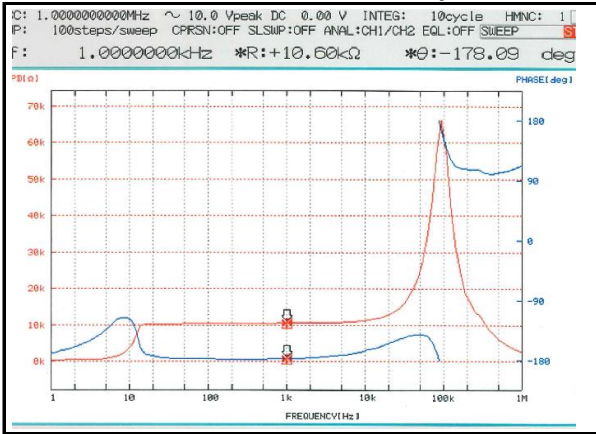
1 L35-89E 10KΩ : 10KΩ の時
