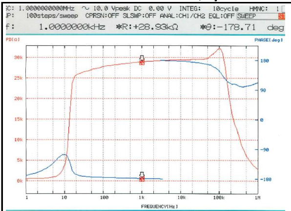
3 L35-89E 30KΩ : 30KΩ の時
