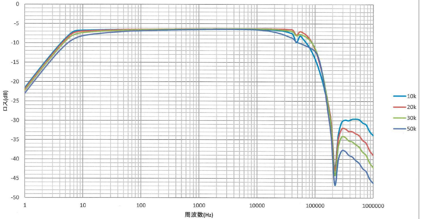
1 L35-89E 10KΩ : 10KΩ の時
