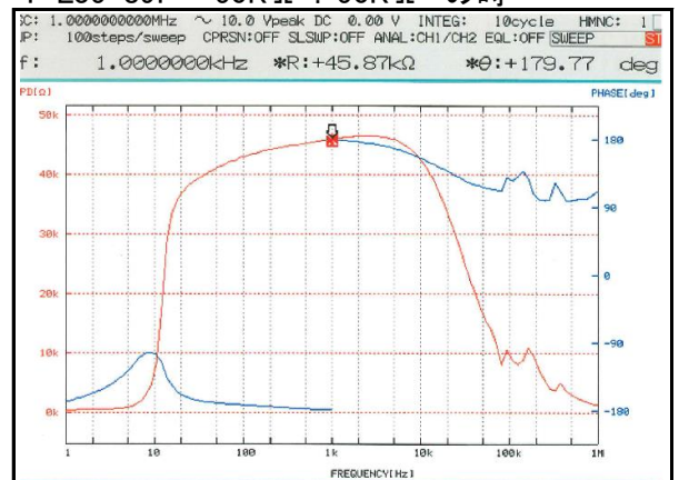
4 L35-89F 50KΩ : 50KΩ の時
