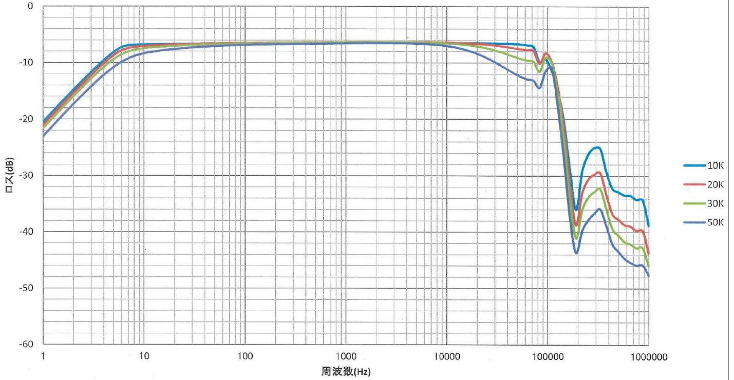
1 L35-89F 10KΩ : 10KΩ の時
