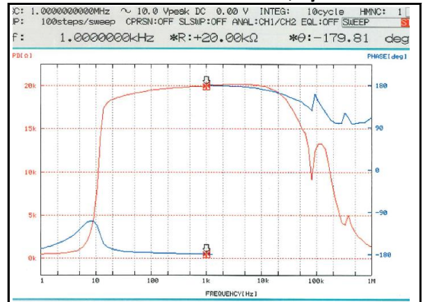
2 L35-89F 20KΩ : 20KΩ の時
