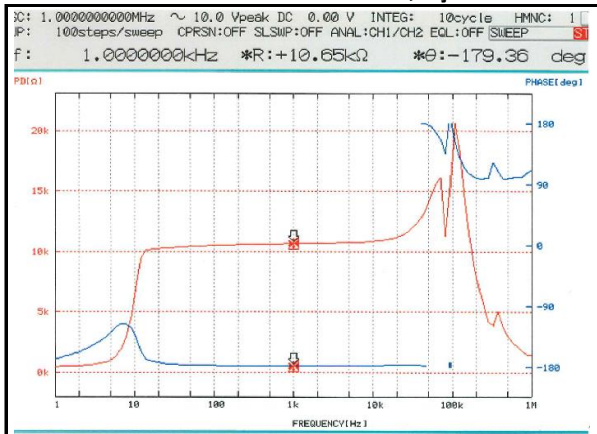
1 L35-89F 10KΩ : 10KΩ の時
