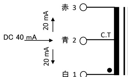
接続図
