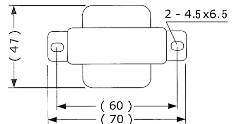
外形寸法図
