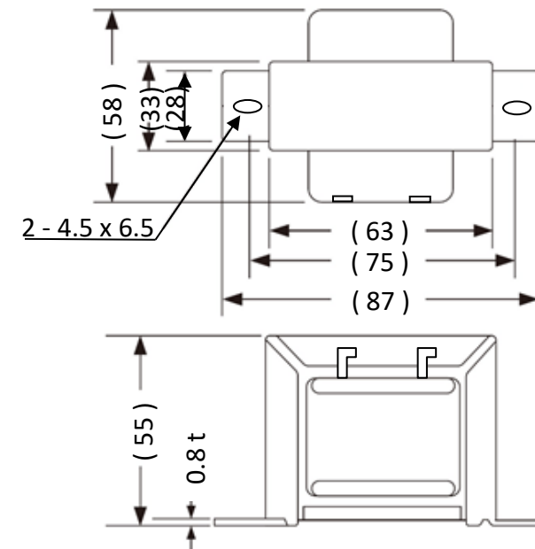
外形寸法図
