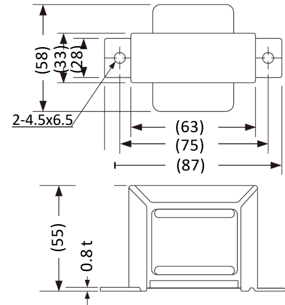
外形寸法図
