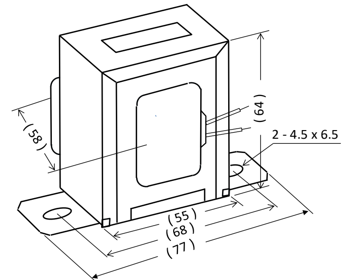
外形寸法図
