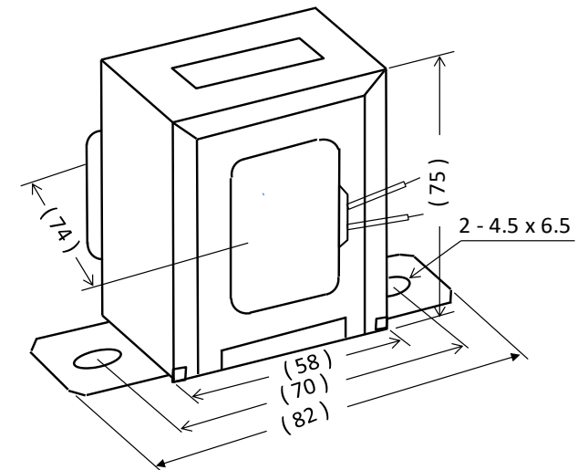
外形寸法図
