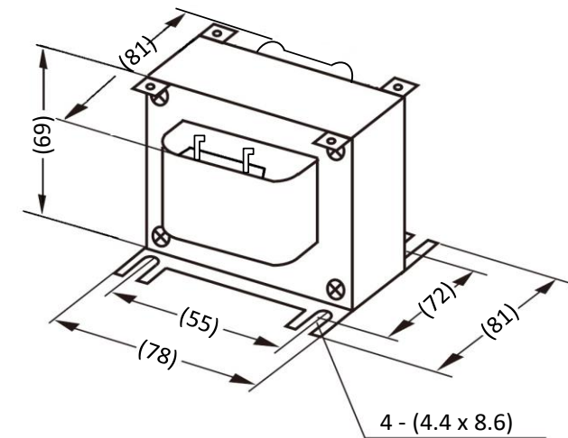
外形寸法図
