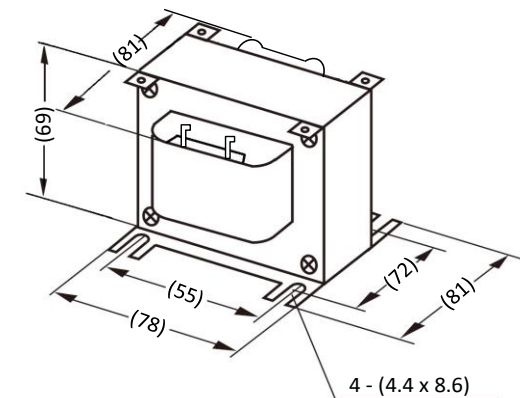
外形寸法図
