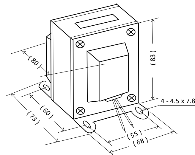
外形寸法図
